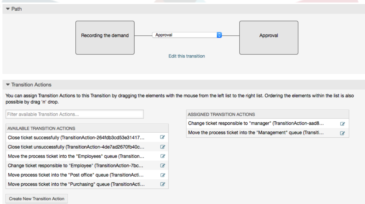
Figure 5.22. Назначить Действия Перехода
